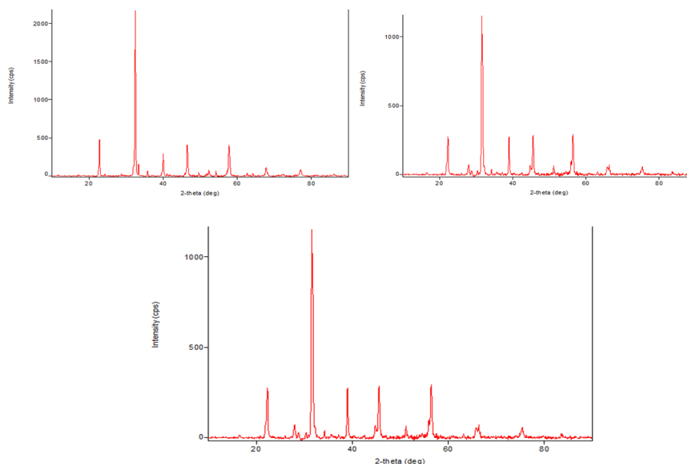
Рисунок 1 – Рентгеновские дифракционные картины образцов
