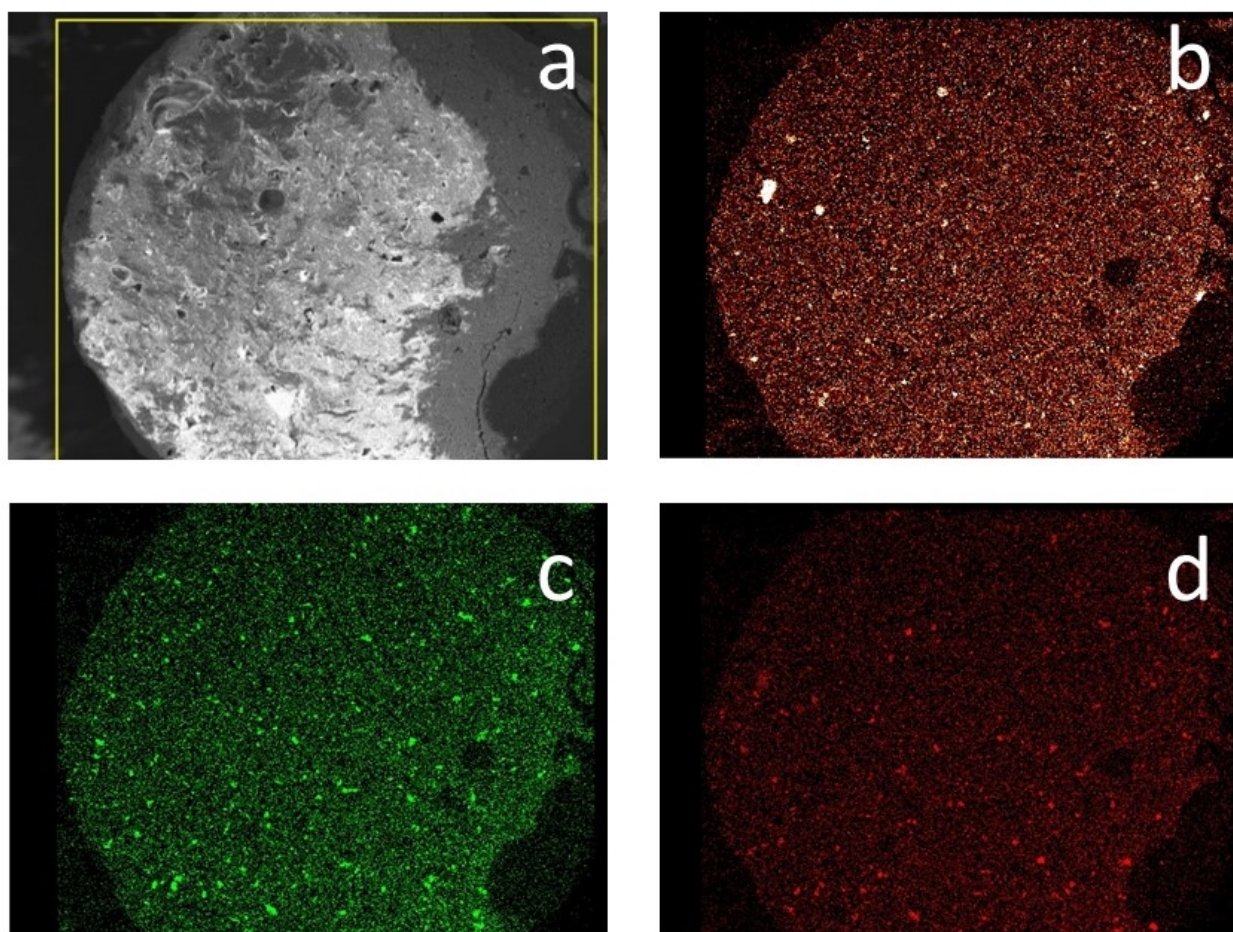
1-сурет. Катализатор түйіршігінің шеткі бетігі бойынша элементтердің таралуы (а. - электрондық микрофотография, б. - Mn, с. - Cr, d. - Fe)
