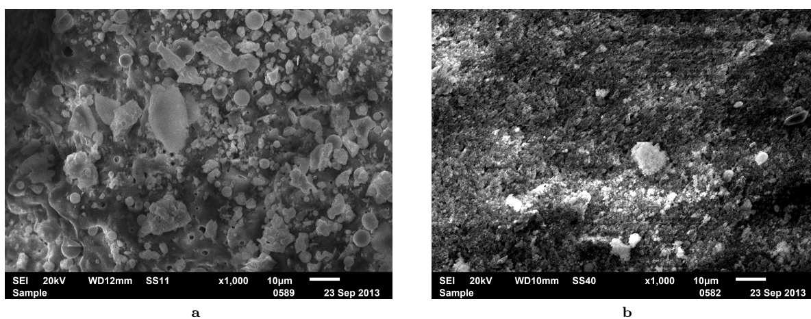
2-сурет. Үлгілердің электронды микрофотографиялары (а. - қалдықтардың бастапқы сынамасы, б. - термоөңделген түйіршіктелген катализатор)
