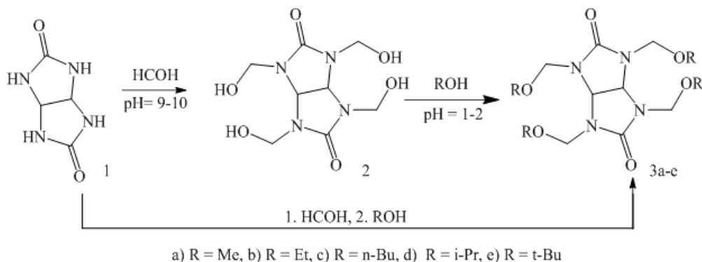
Схема 1 – Синтез тетра(алкоксиметил)гликолурилов 3а-е
